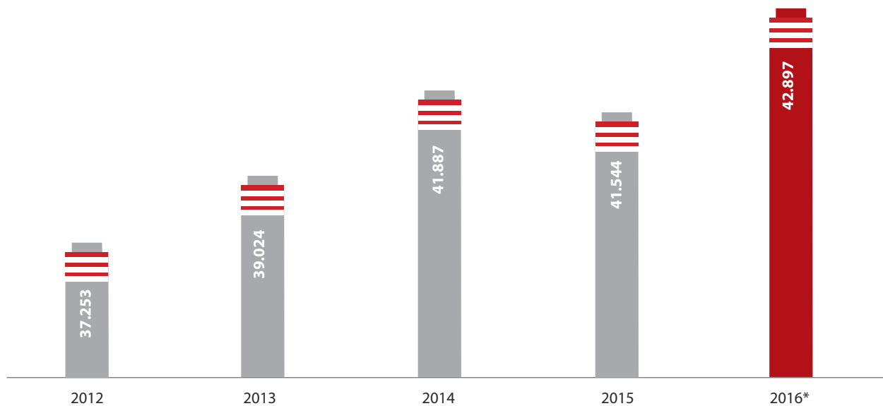
Grafik Daya Mampu Netto (DMN) Pembangkit di Indonesia Tahun 2012-2016 (MW)
